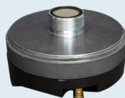
DR 10 PRO PVP 39,00€ MARK 80hm Motor de compresión. 40 W @ 8 Ohm. Rosca 35 mm.
